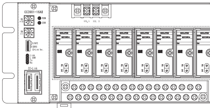
図 13.4. 取付け姿勢
