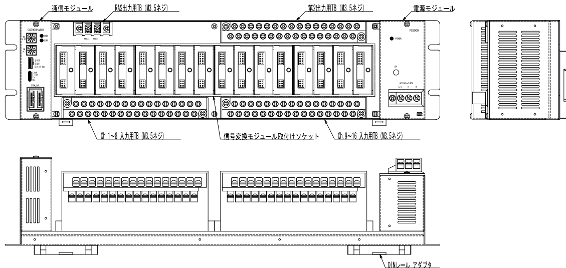
図 4.1. CC3901-16AI 全体構成図
