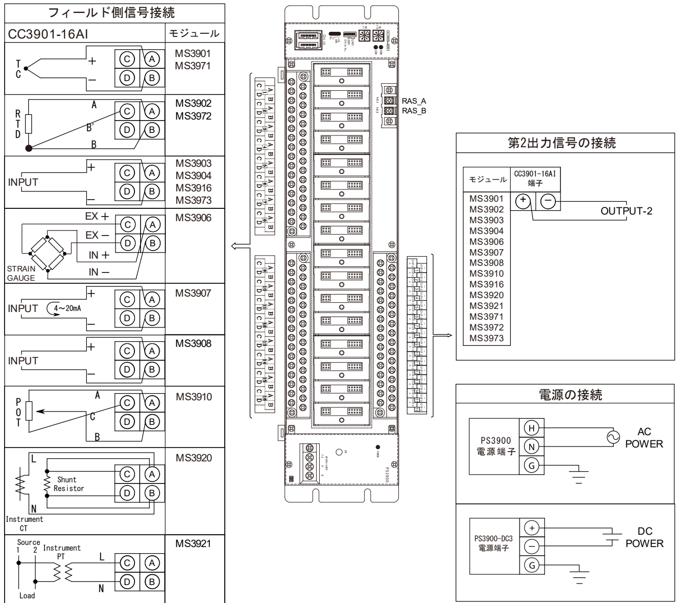
図 9.1. 入出力信号及び電源の接続図
