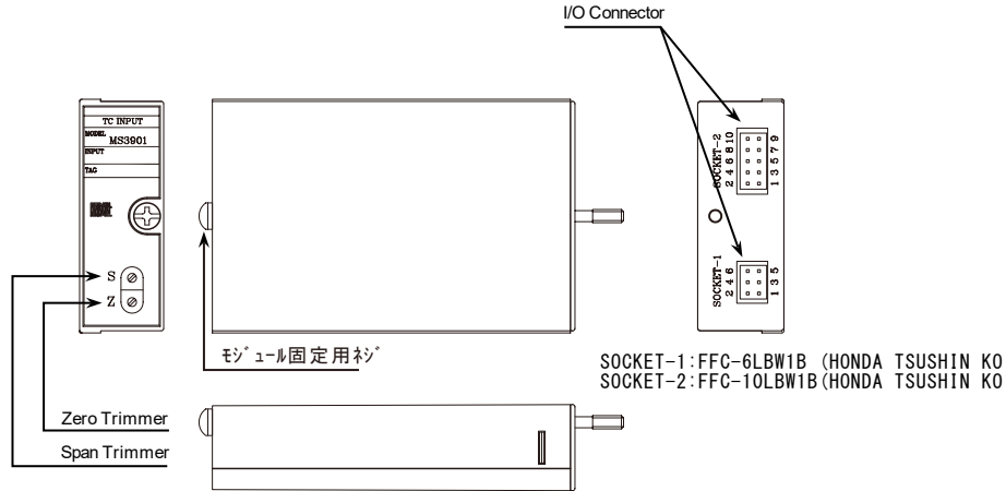
図 5.2. 信号変換モジュール外観図
