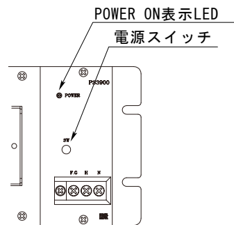
図 5.1. 電源モジュール外観図
