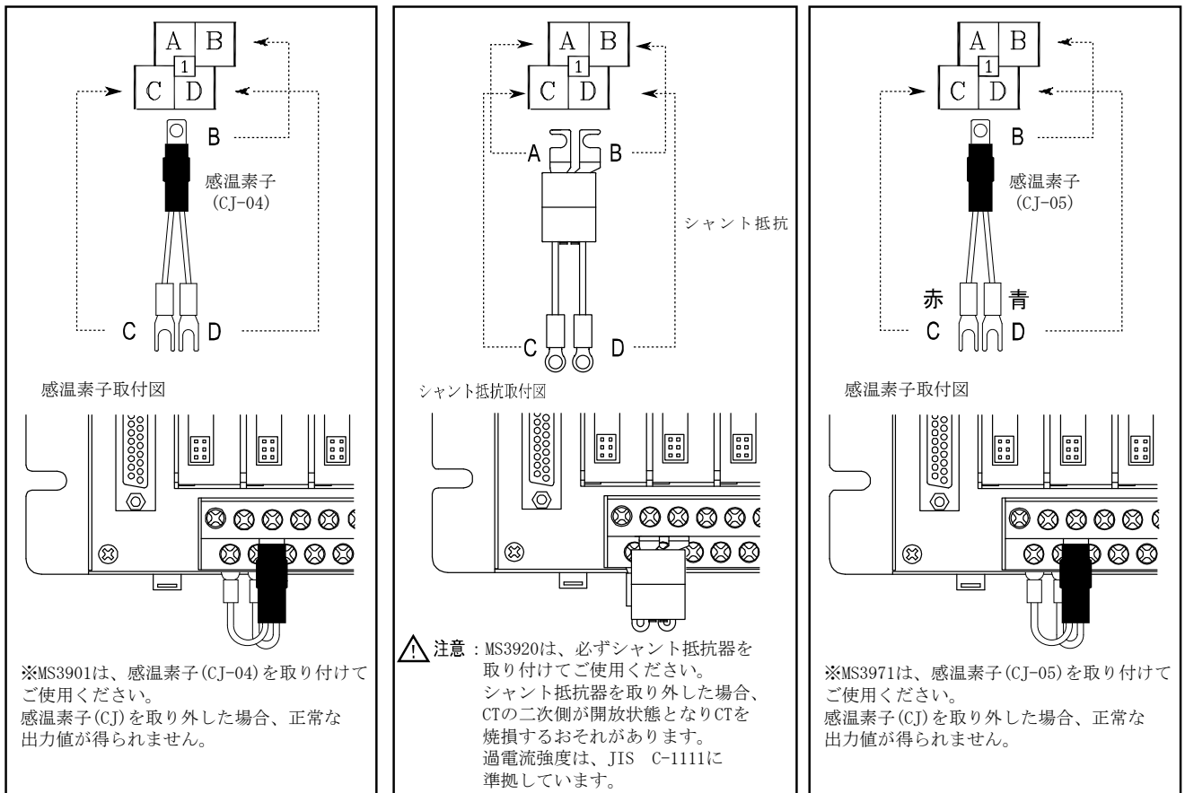
図 5.3. MS3901、MS3920、MS3971 接続図
