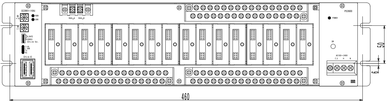
図 13.2. 壁取付け
