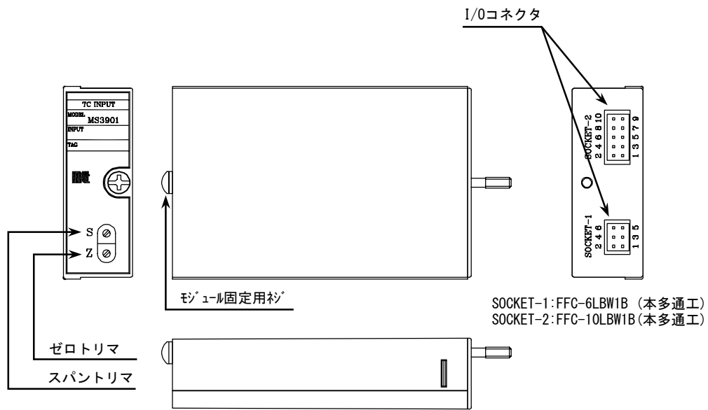
図 5.2. 信号変換モジュール外観図
