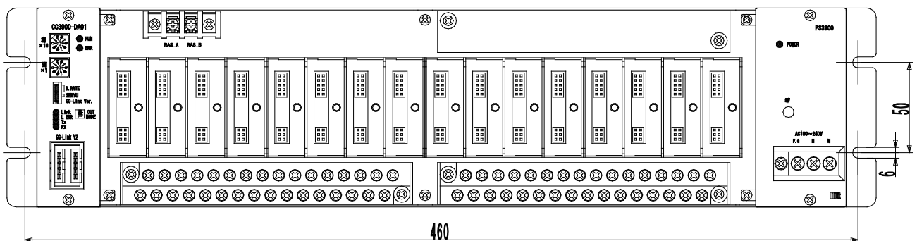
図 12.2. 壁取付け
