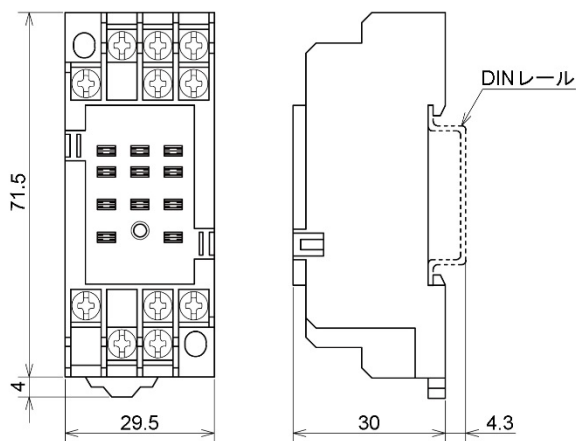
11P ソケット(MGBW)
