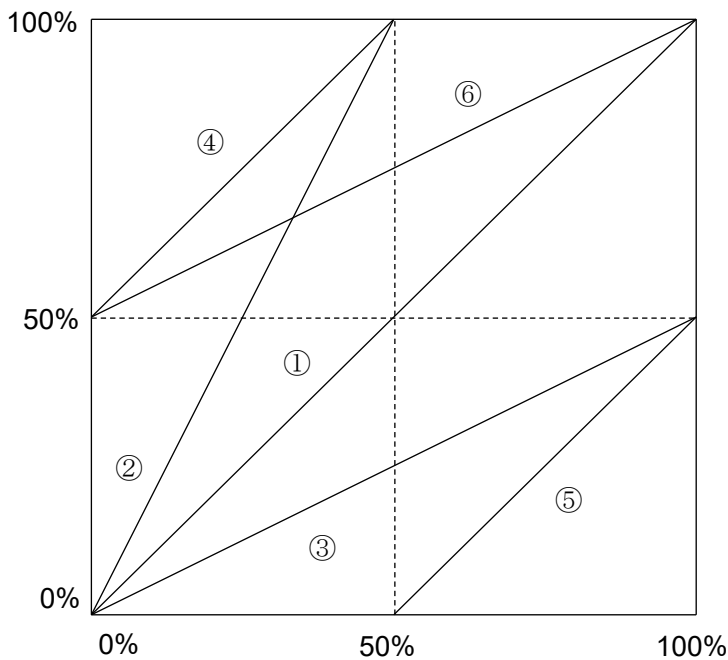
(図8.2-1 ノーマル出力時)
