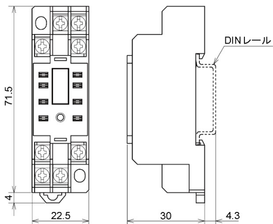
8P ソケット(MGB, MGBL)
