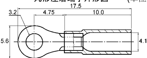
丸形圧着端子外形図
