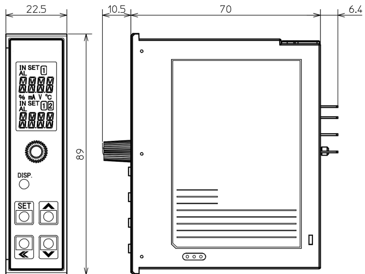
8P ソケット(MGF, MGFL)
