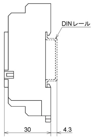
11P ソケット(MGIW)
