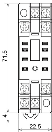
8P ソケット(MGI, MGIL)
