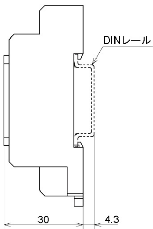
8P ソケット(MGI, MGIL)
