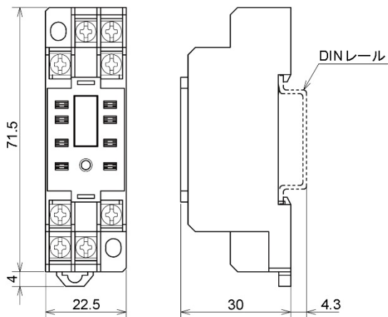
8P ソケット(MGI, MGIL)
