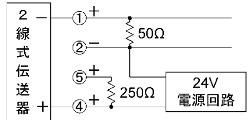
(図4.4-4) 2出力(入力抵抗約50Ω)
