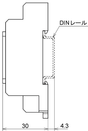
8P ソケット(MGS, MGSL)
