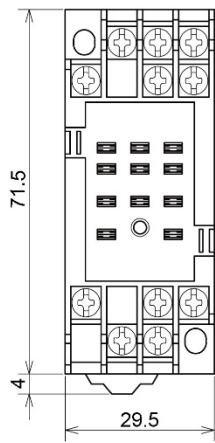
11P ソケット(MGSW)
