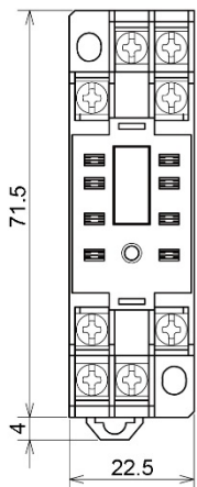
8P ソケット(MGS, MGSL)
