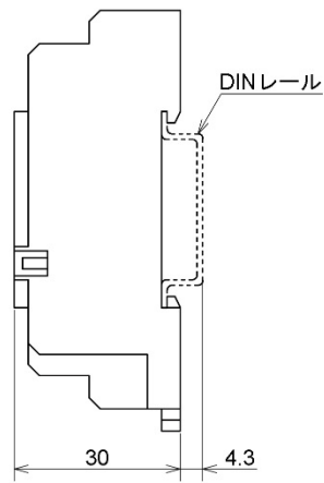
11P ソケット(MGSW)
