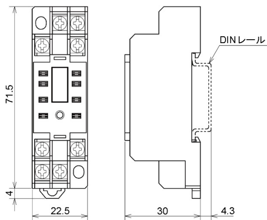
8P ソケット(MGS, MGSL)
