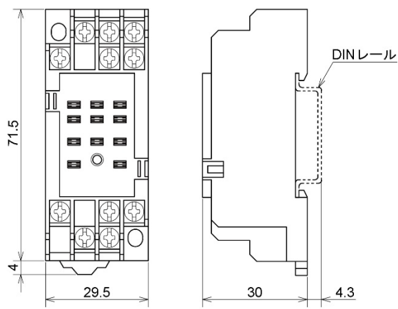
11P ソケット(MGSW)
